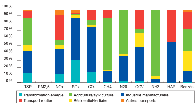
Émissions en Nord-Pas-de-Calais en 2005. (Source Atmo Nord Pas-de-Calais)
